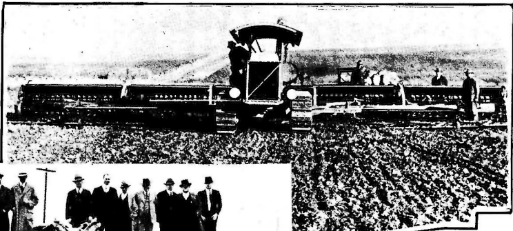
LA MAYOR MAQUINA SEMBRADORA del mundo es este gigantesco aparato, construido por F. W. Schwardt para una granja de Idaho, Estados Unidos. Con este aparato pueden sembrarse 150 acres en diez horas.
